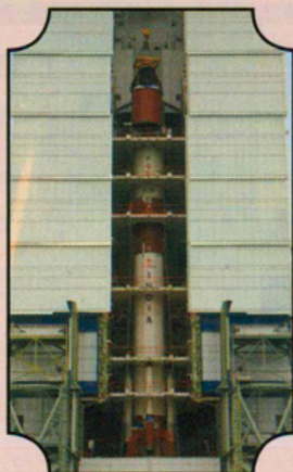
PS3-PS4 Module Stacking
